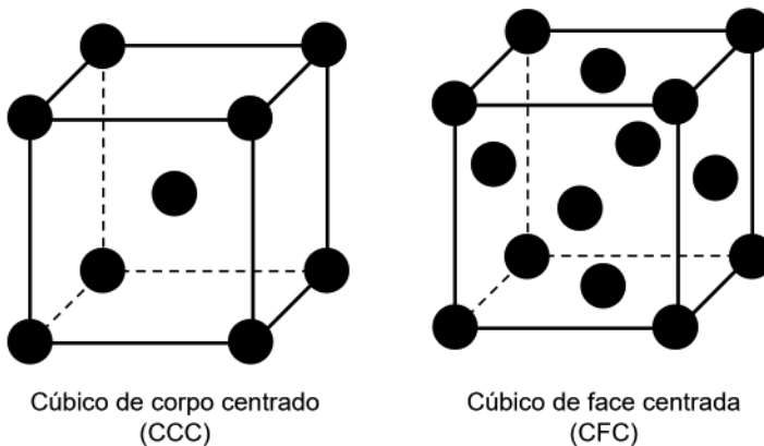
Figura 1.1 – Reticulados cristalinos do ferro. Fonte: adaptada de (1).
