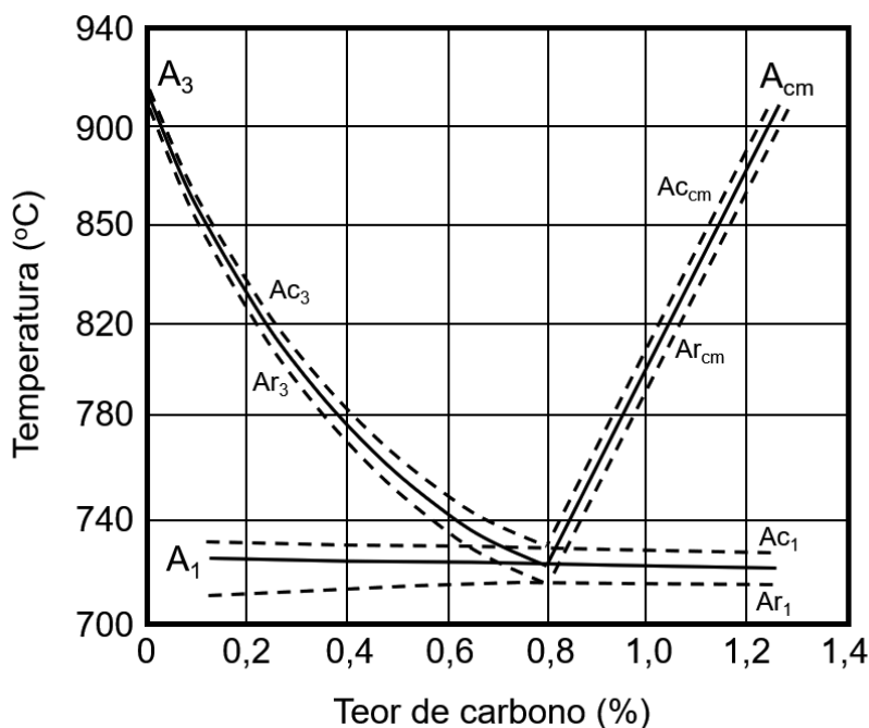
Figura 1.8 – Efeito do resfriamento e do aquecimento nas temperaturas de transformação alotrópica. Fonte: adaptada de (7).
