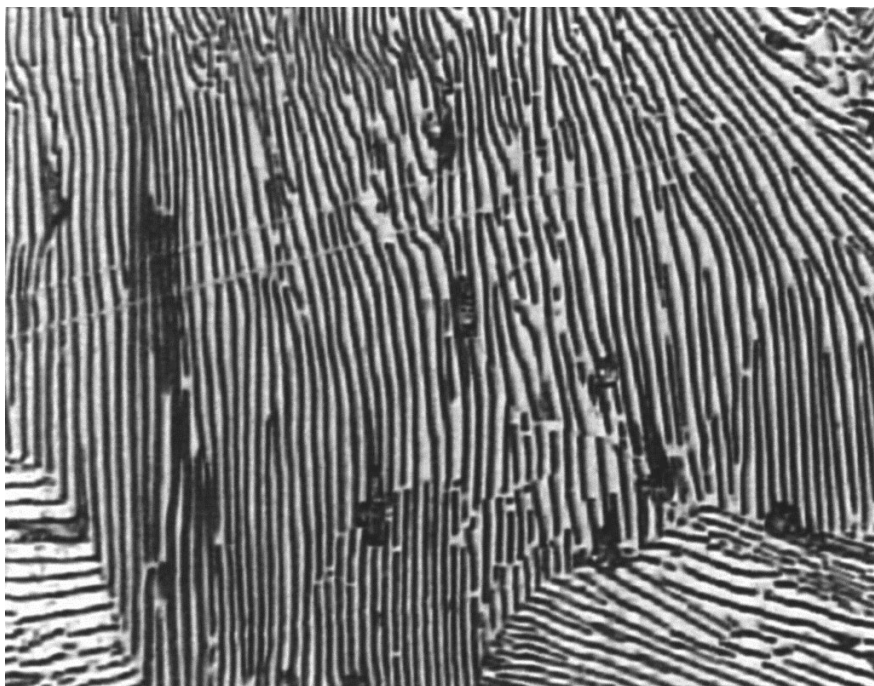
Figura 1.7 – Microestrutura da perlita na composição eutetoide. Nital 2%. 500x. Fonte: o autor.
